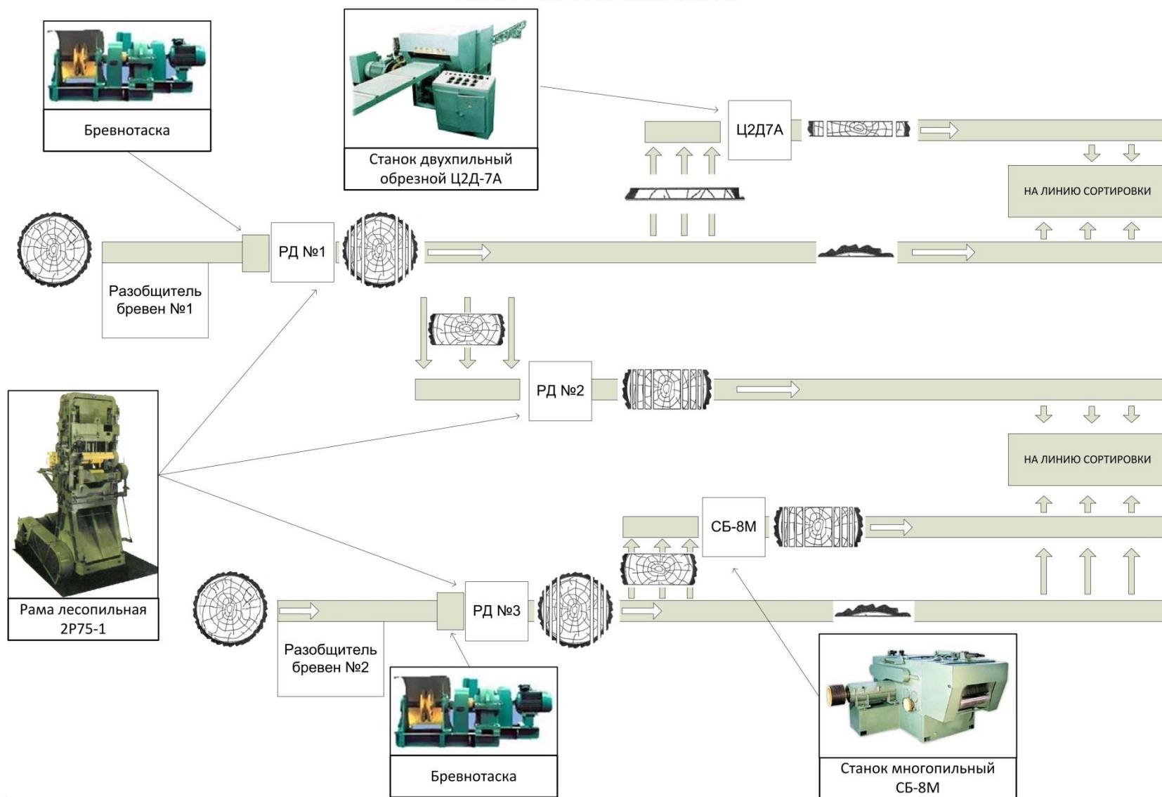
СХЕМА УЧАСТКА ЛЕСОПИЛЕНИЯ
